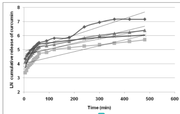
Fig. 4: First-order drug release kinetic (F1 (-■-); F2 (-▲-); F3 (-x-); F4 (-◆-))
