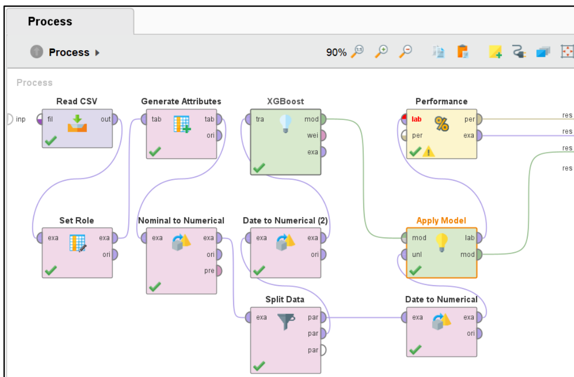
Gambar 3. Implementasi Algoritma XGBoost
