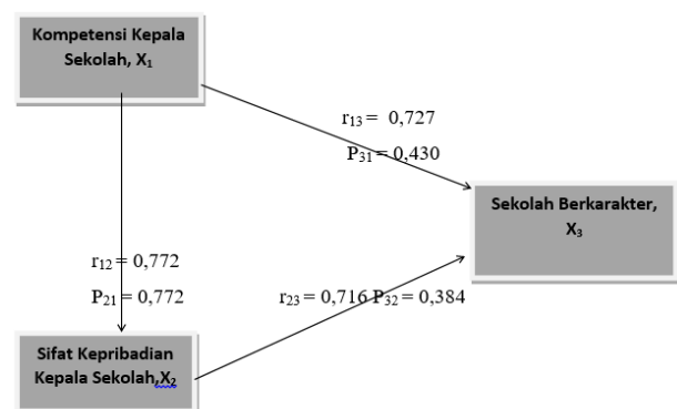
Gambar 1. Model Diagram Jalur Hasil Pengujian
