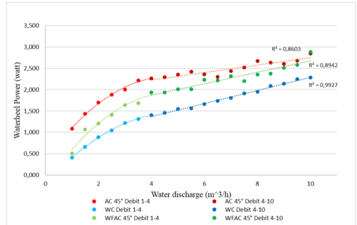
Fig. 6. Waterwheel Power (watt)
