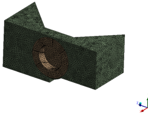
Fig. 6. Global Meshing
