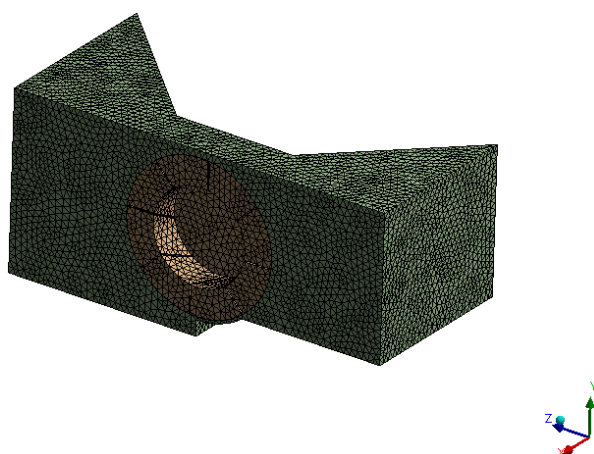
Fig. 6. Global Meshing
