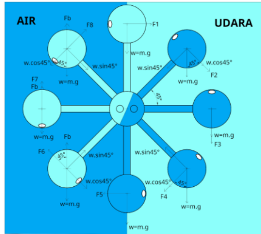
Gambar 3. Gaya-Gaya Yang Bekerja Pada Kincir Bouyancy
