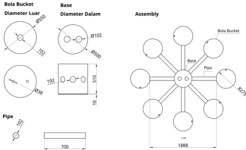
Gambar 2. Skema Uji Kincir Bouyancy
