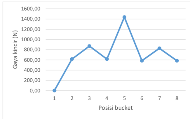
Gambar 4. Grafik Gaya Ember Bola
