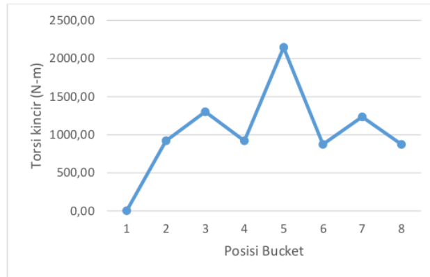
Gambar 5. Grafik Gaya Torsi
