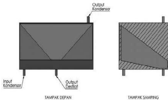
Gambar 2 Kondensator
