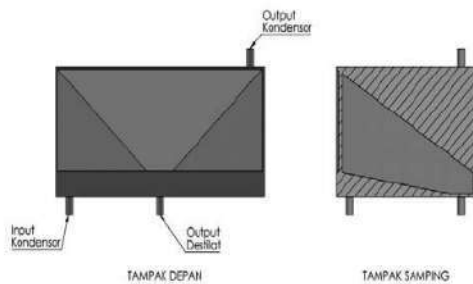
Gambar 2 Kondensator
