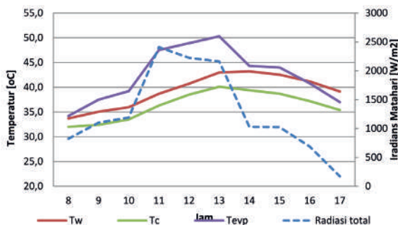
Gambar 5 Grafik temperatur solar still Seperti di tampilan pada Gambar 5, temperatur evaporasi atau temperatur uap lebih
