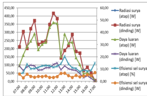
Gambar 2. Distribusi Kinerja Panel Surya (Utara)
