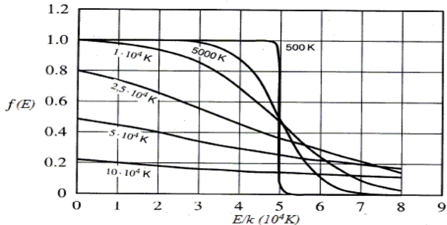
Gambar 5 Energi Fermi
