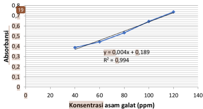
Gambar 8. Kurva Kalibrasi Asam Galat
