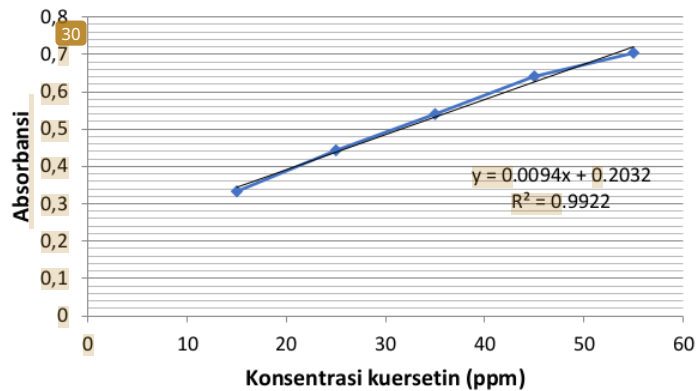
Gambar 7. Kurva Kalibrasi Kuersetin
