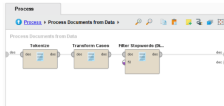
Gambar 4. Operator yang digunakan dalam process document
