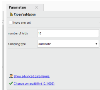
Gambar 7. Parameter cross validation yang digunakan
