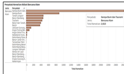
Gambar 7. Grafik Penyebab Kematian Akibat Bencana Alam
