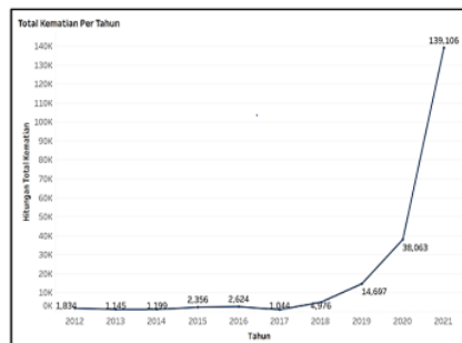
Gambar 9. Grafik Total Kematian Per Tahun
