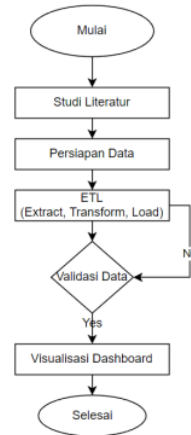
Gambar 1. Langkah-Langkah Penelitian
