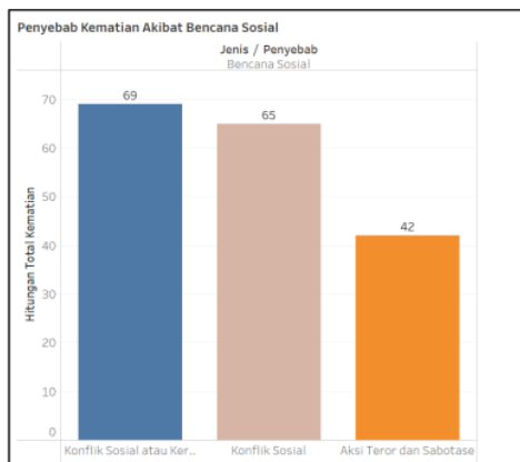
Gambar 6. Grafik Penyebab Kematian Akibat Bencana Sosial
