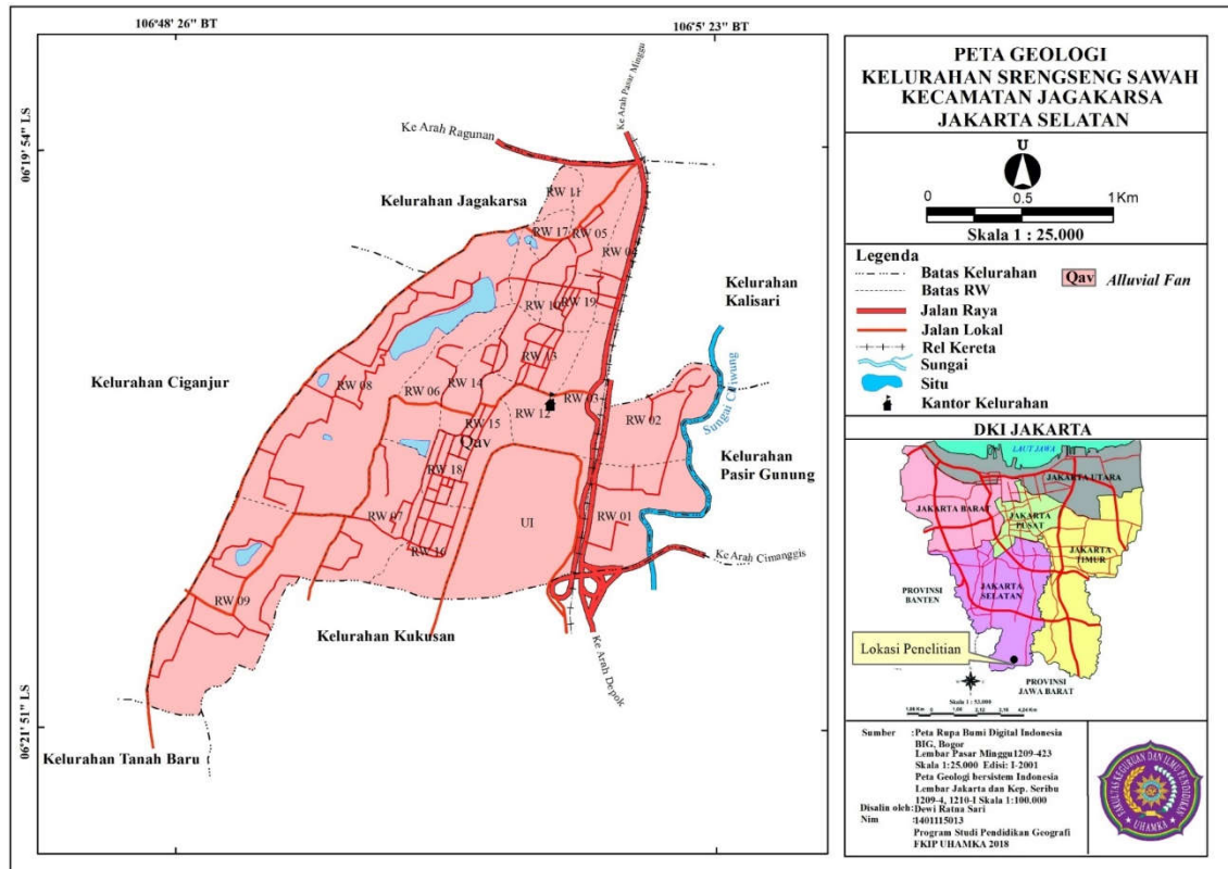
Peta 2 Peta Geologi Kelurahan Srengseng Sawah
