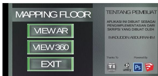
Gambar 5 inteface aplikasi
