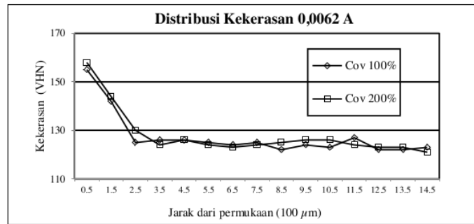
Gambar 3. Distribusi kekerasan setelah di shot peening 0.0062 A
