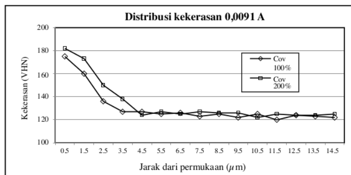
Gambar 4. Distribusi kekerasan setelah di shot peening 0.0091 A
