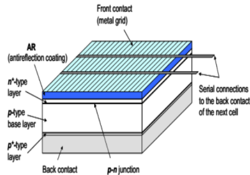
Gambar 2 Tipikal Struktur Sel surya
