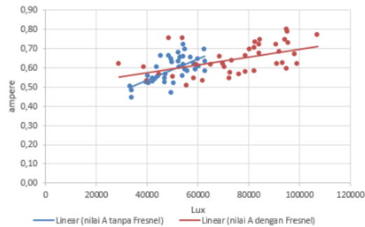
Gambar 9 Grafik Intensitas Radiasi dengan Arus yang di dapat
