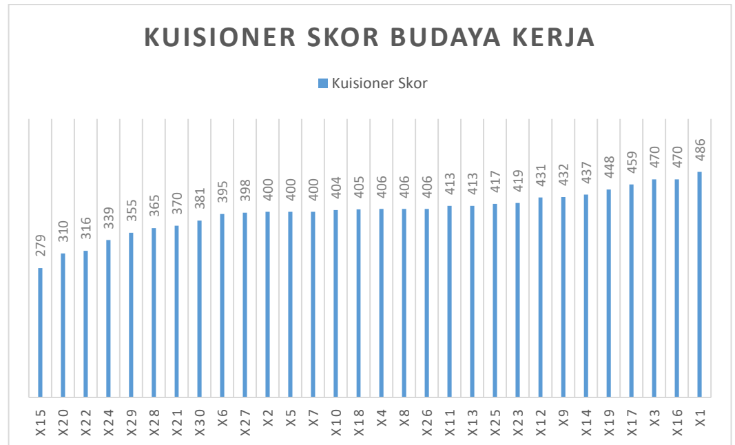
Gambar 5 Histogram Kuisisioner Skor Budaya Kerja
