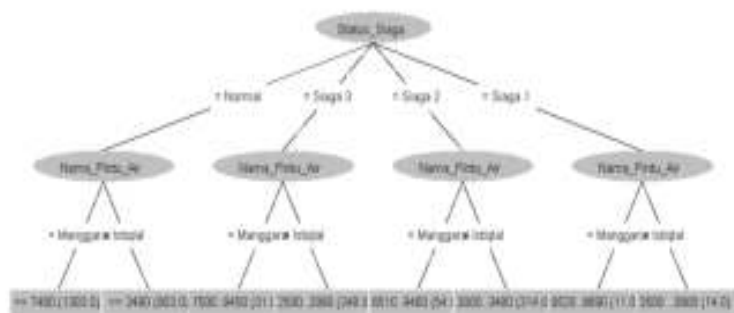
Gambar 4 Visualisasi hasil model decision tree yang berbetuk
