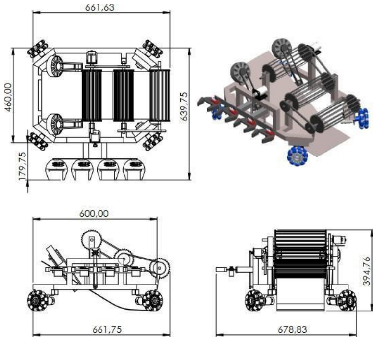
Gambar 3. Desain Mekanik Forklift Robot
