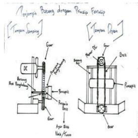
Gambar 2. Desain Mekanik Forklift Robot.
