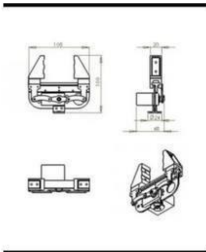
Gambar 1. Desain Mekanik lengan Robot.
