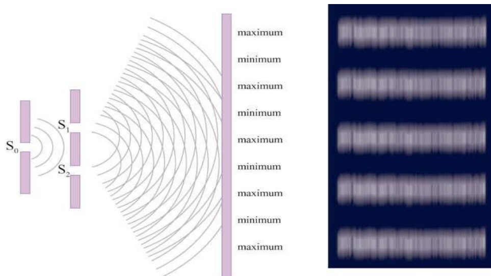
Gambar 1. Pola gelap terang hasil interferensi celah ganda
