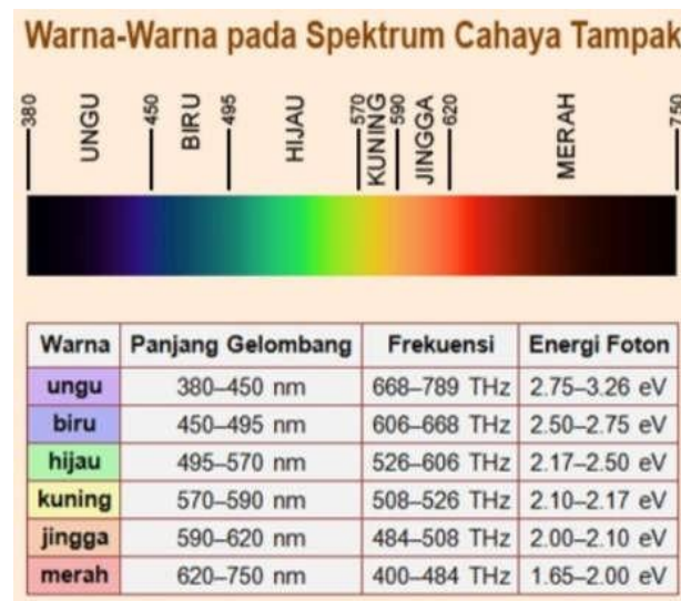
Gambar 3. Spektrum cahaya tampak
