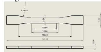
Gambar 3.1 Ukuran spesimen ASTM-D638
