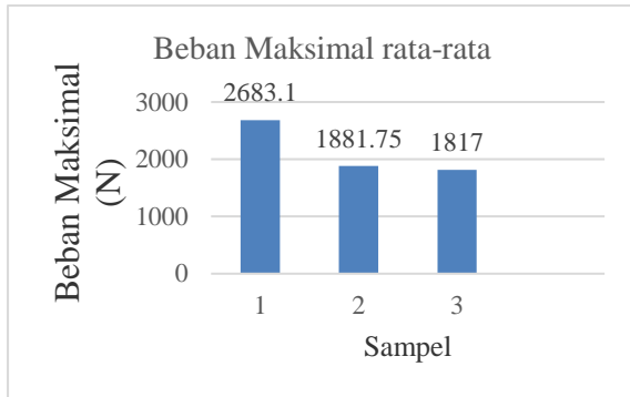
Gambar 4.2 Grafik nilai rata-rata Fmax
