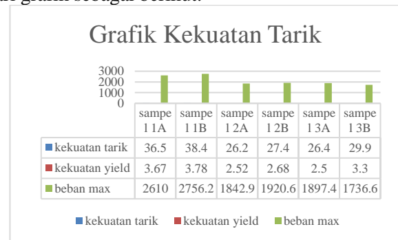
Gambar 4.1 Grafik pengujian tarik
