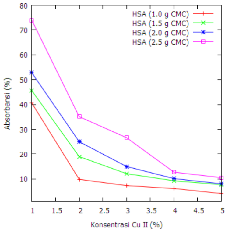
GAMBAR 1. Kurva serapan ion logam Cu (II)
