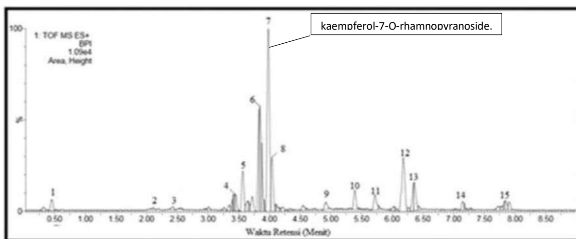
Gambar 9.6. Kromatogram LC-MS Ekstrak Etanol 70% Daun A. conyzoides (Tambunan et al., 2014)
