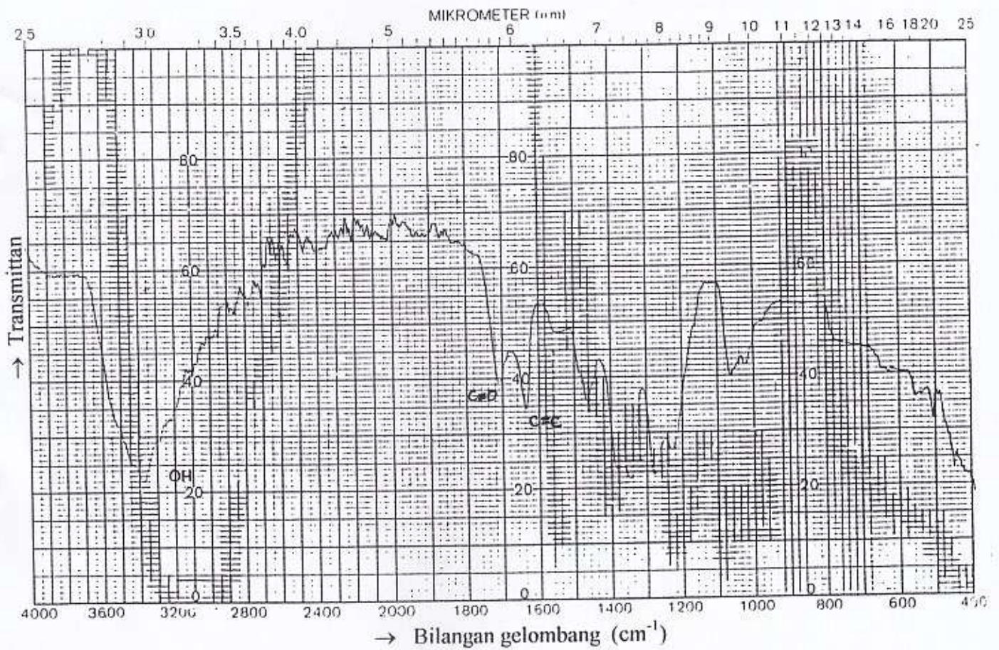
Gambar 12. Spektrum Inframerah Senyawa V-1
