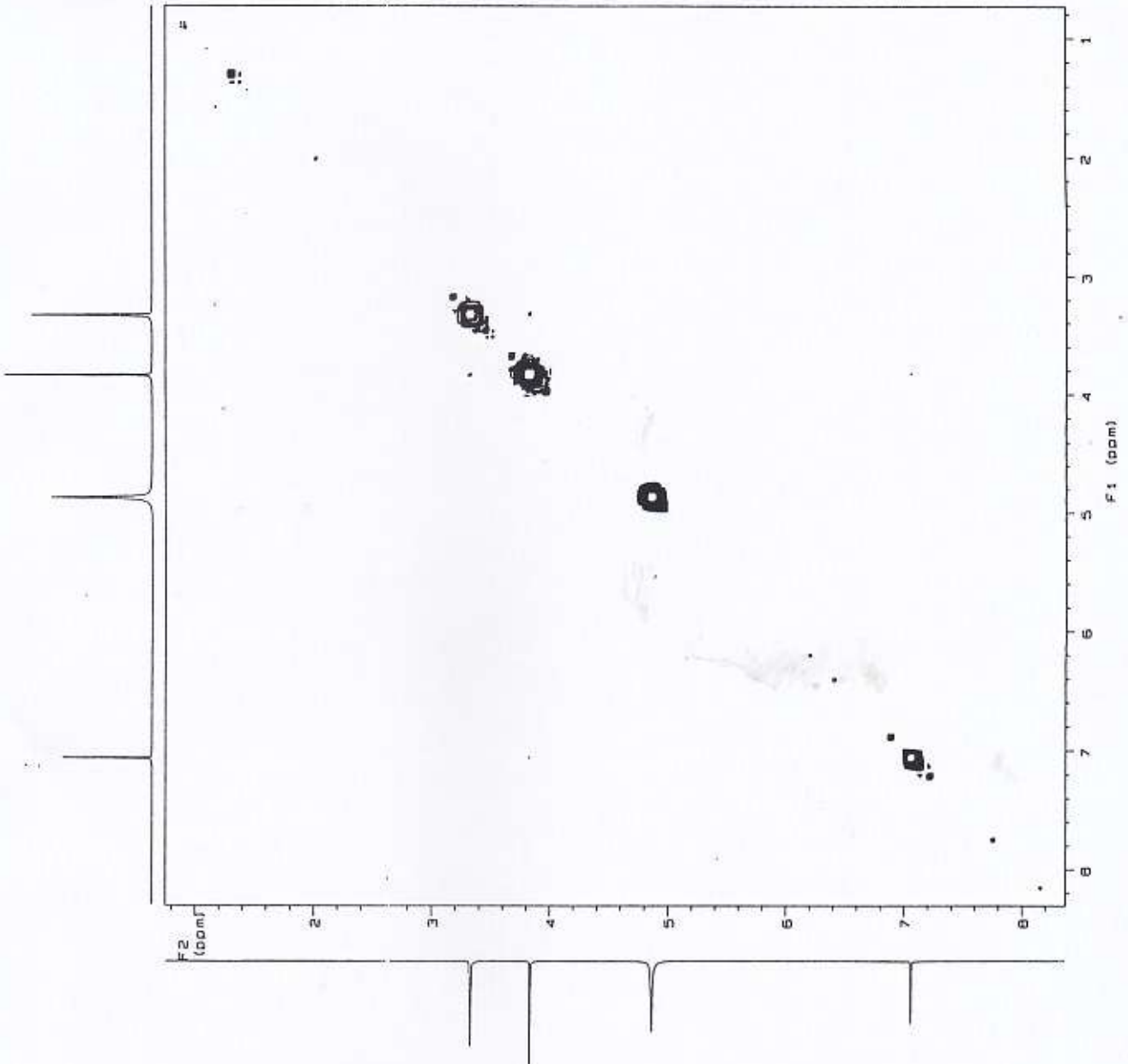
Lampiran 20. Spektrum COSY Senyawa V-1 dalam CD 3 OD
