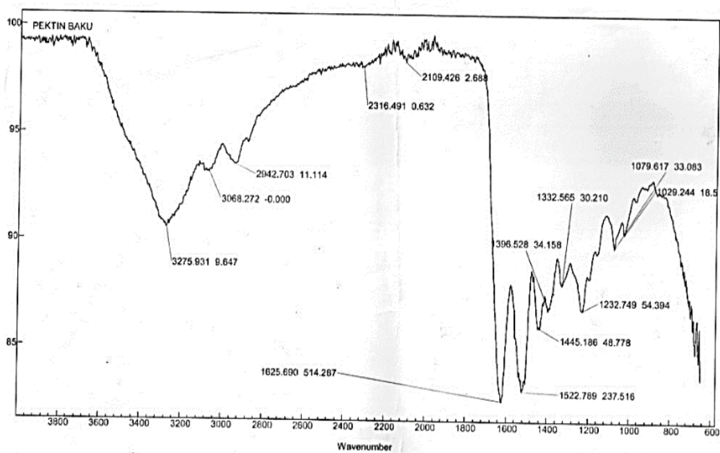
Gambar 1. Hasil spektrum IR pektin baku
