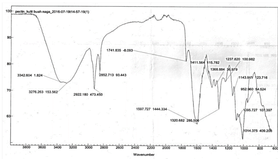
Gambar 2. Hasil spektrum IR pektin kulit buah naga merah
