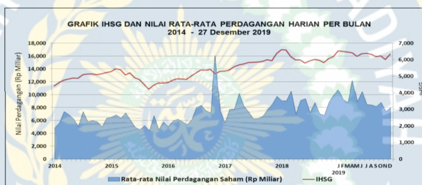
Gambar 1 Perkembangan IHSG 2014-2019
