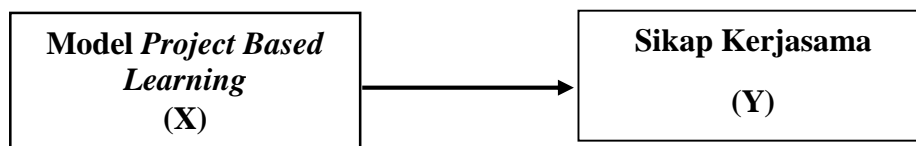
Gambar 2.1 Kerangka Berfikir
