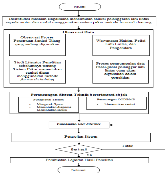
Gambar 3 Metodologi Penelitian
