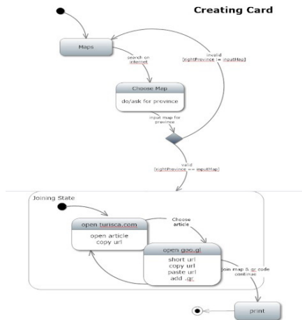
Gambar 7 State Diagram Pembuatan Kartu
