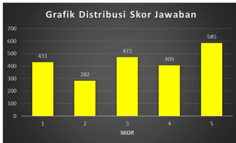
Gambar.1 Grafik Distribusi Skor Jawaban
