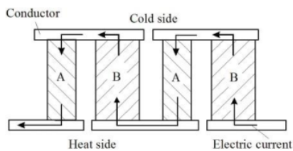
Gambar 1. Generator termoelektrik[15]
