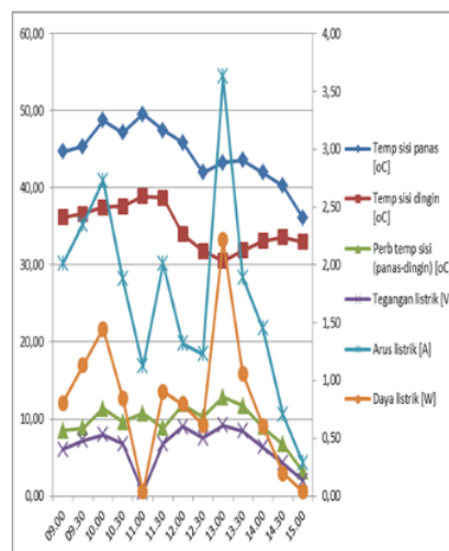
Gambar 2. Distribusi hasil pengukuran pada susunan seri TEG
