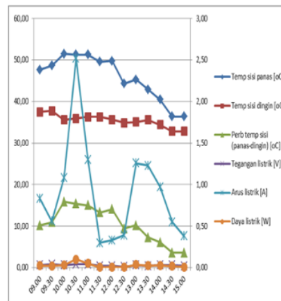
Gambar 3. Distribusi hasil pengukuran pada susunan paralel TEG
